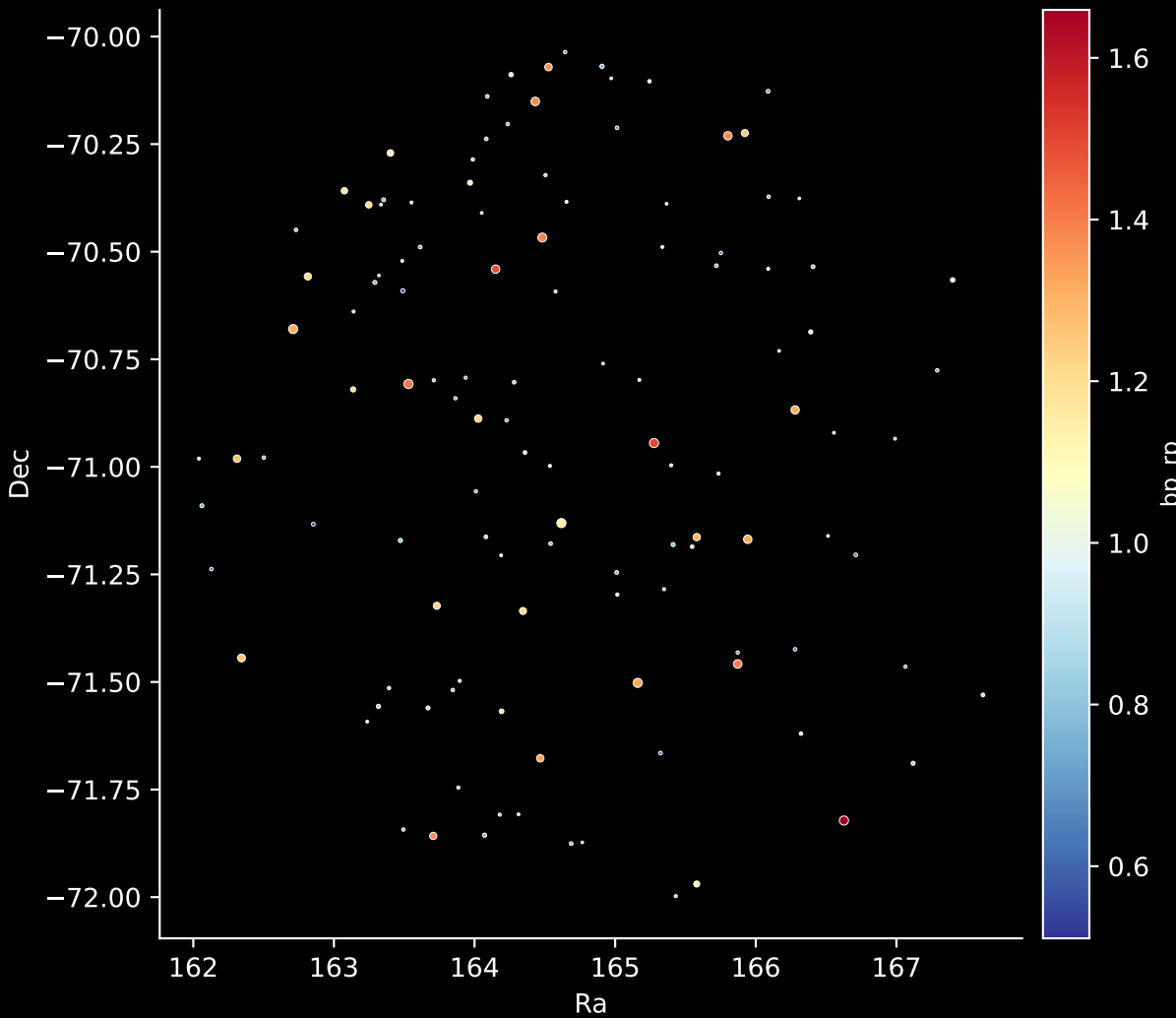
GALAH DR4 Field: [7207] Stars: 119
