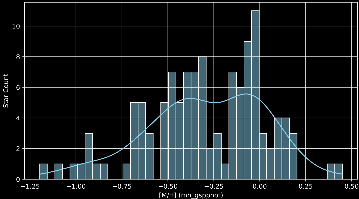
GALAH DR4 Field: [7207] [M/H] (mh_gspphot) (n= 119)
