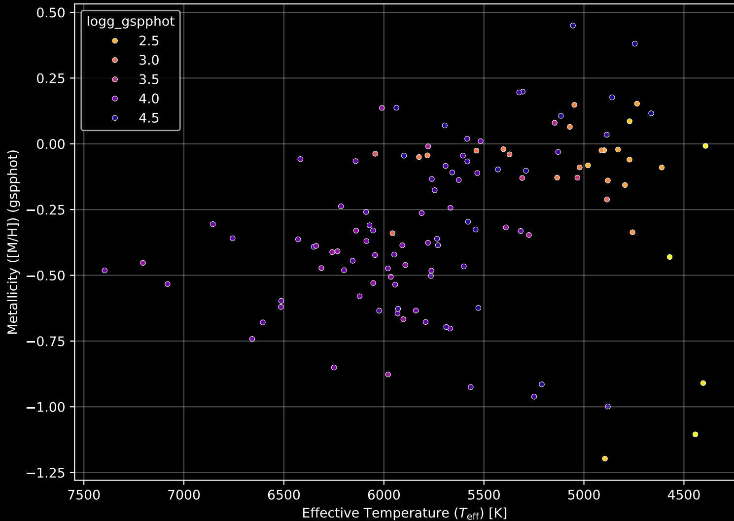
GALAH DR4 Field: [7207] Stellar Population Parameters (n= 119)
